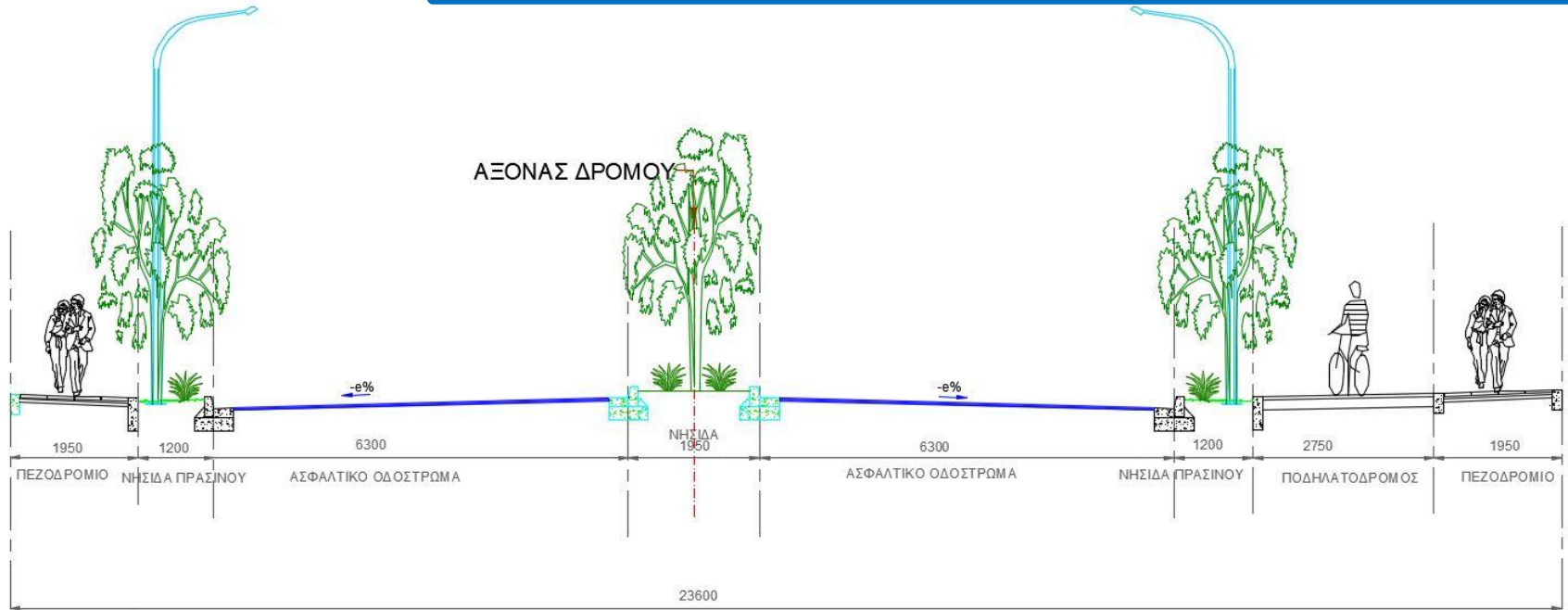
ΤΥΠΙΚΗ ΔΙΑΤΟΜΗ- Δρόμος Πρωταρχικής Σημασίας (Τμήμα που συνδέει τη Λεωφ. Στροβόλου με τη Λεωφ. Αρχαγγέλου)
