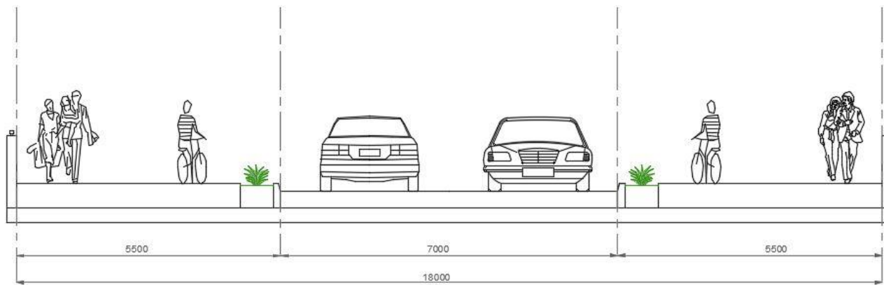
διατομή οδοστρώματος γέφυρας 2
